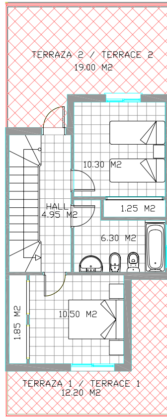
PLANTA PRIMERA FIRST FLOOR
