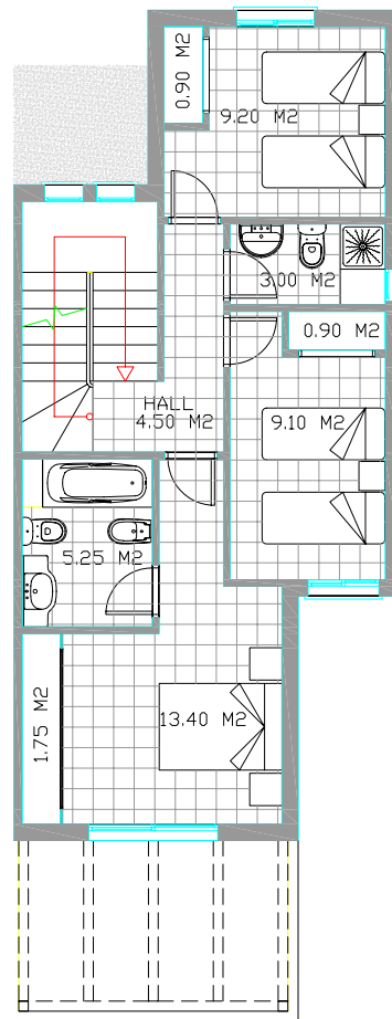
PLANTA PRIMERA FIRST FLOOR
